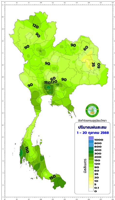
ปริมาณฝนสะสม 1-20 ตุลาคม 2568
