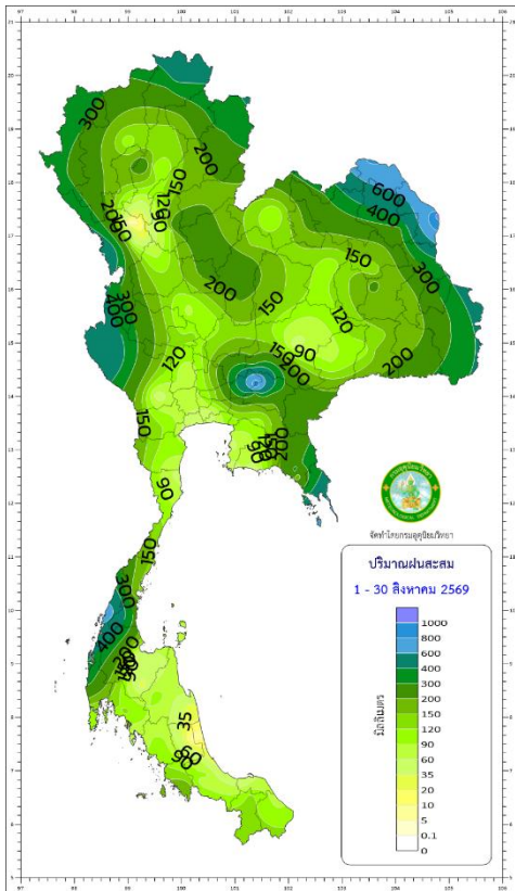
ปริมาณฝนสะสม 1-30 สิงหาคม 2569
