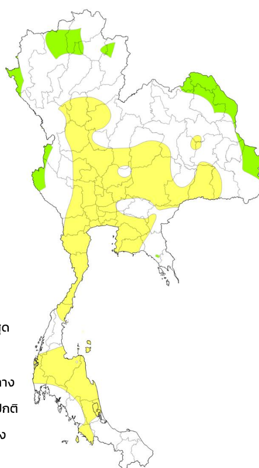
7 วันข้างหน้า (9 – 15 มิ.ย. 68)
