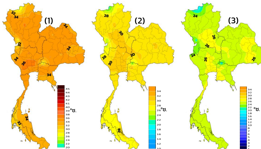
(1)อุณหภูมิสูงสุดเฉลี่ย (2)อุณหภูมิเฉลี่ย (3)อุณหภูมิต่ำสุดเฉลี่ย ระหว่างวันที่ 2 - 8 มิ.ย. 68
