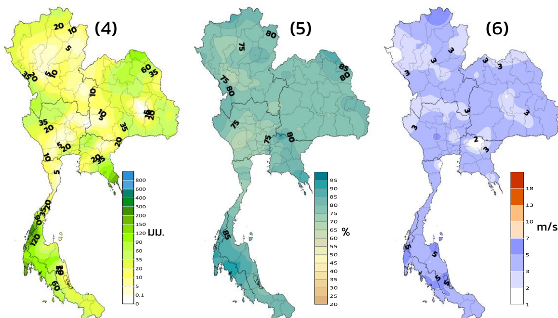
(4)ปริมาณฝนสะสม (5)ความชื้นสัมพัทธ์ (6)ความเร็วลมสูงสุดเฉลี่ย ระหว่างวันที่ 2 - 8 มิ.ย. 68
