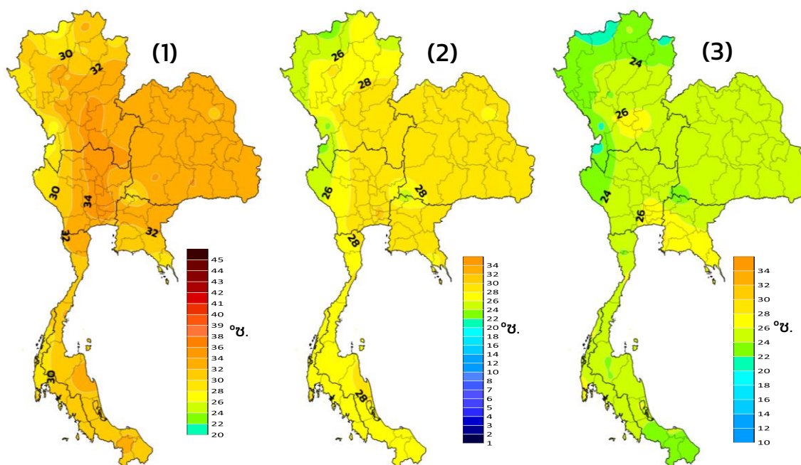
(1)อุณหภูมิสูงสุดเฉลี่ย (2)อุณหภูมิเฉลี่ย (3)และอุณหภูมิต่ำสุดเฉลี่ย ระหว่างวันที่ 9 - 15 มิ.ย. 68
