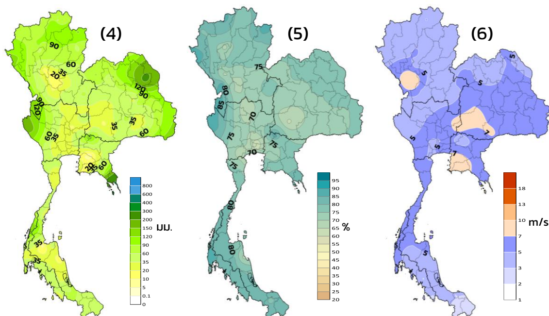
(4)ปริมาณฝนสะสม (5)ความชื้นสัมพัทธ์เฉลี่ย (6)ความเร็วลมสูงสุดเฉลี่ย ระหว่างวันที่ 9 - 15 มิ.ย. 68
