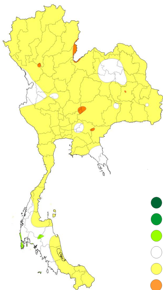
7 วันที่ผ่านมา (2 – 8 มิ.ย. 68)
